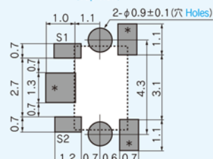
推奨はんだ付けパターン Recommendable soldering pattern (Top view)
